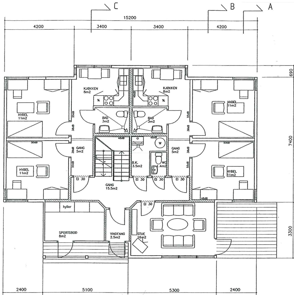
PLAN 1. ETASJE
