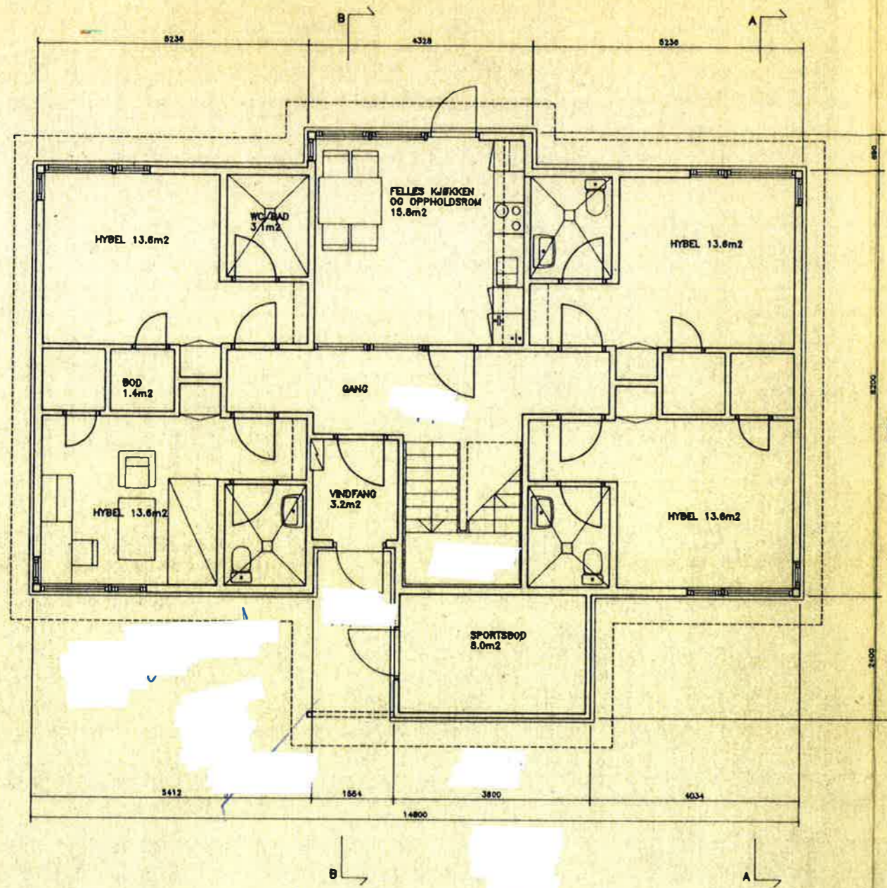
PLAN 1.ETASJE
