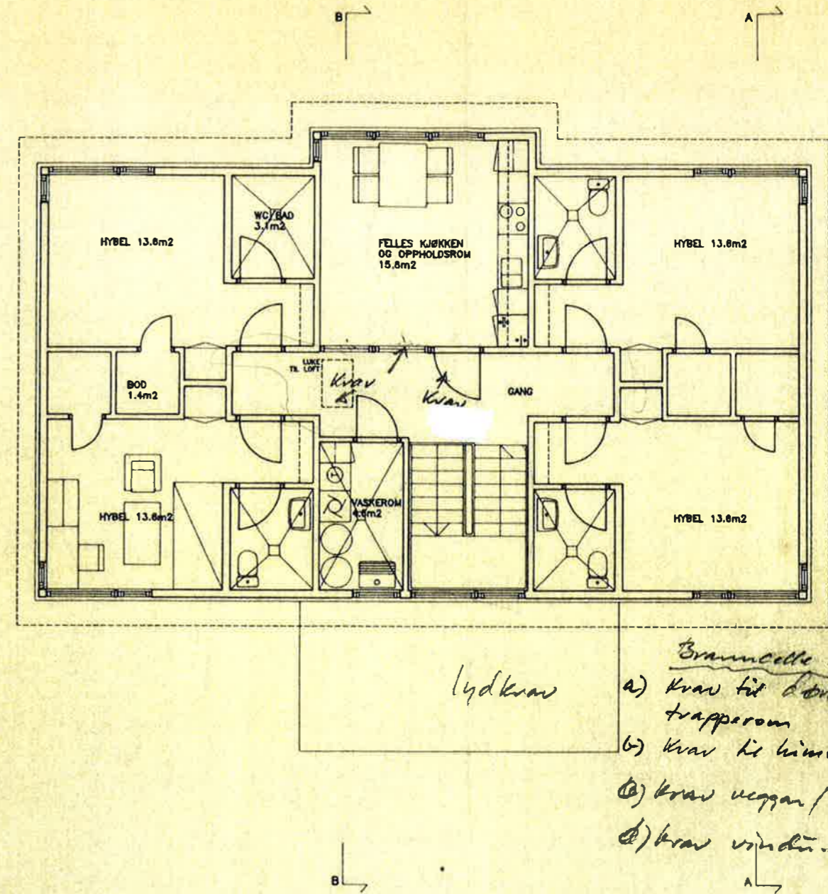
PLAN 2.ETASJE
