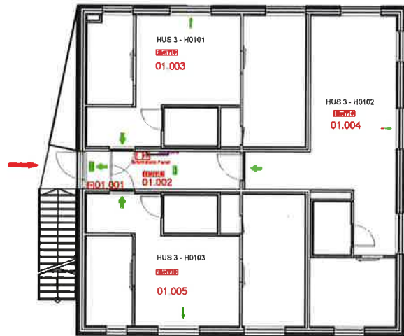
ORIENTERINGSPLAN - FAMILIE 1. ETG.
