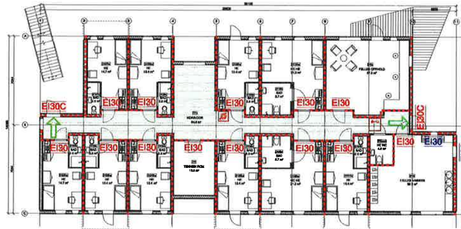
PLAN 1. ETASJE
