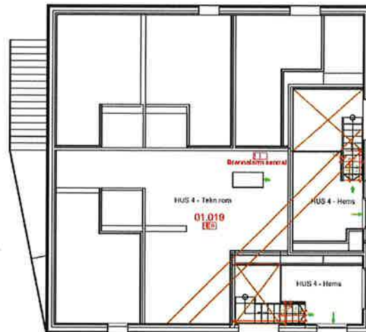
ORIENTERINGSPLAN -ENKLETT HEMS-ETG.
