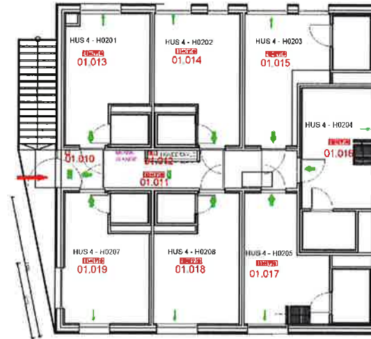
ORIENTERINGSPLAN -ENKLETT 2. ETG.
